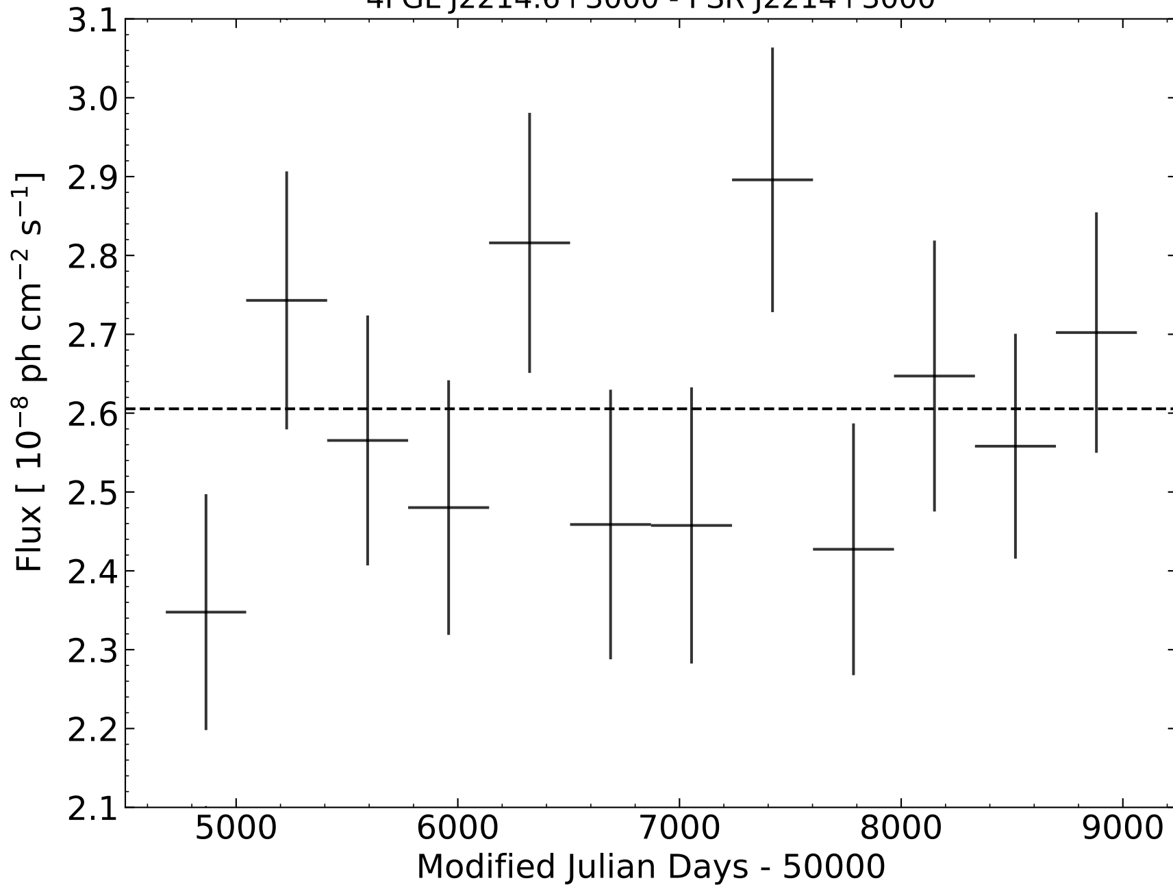
4FGL J2214.6+3000 - PSR J2214+3000
