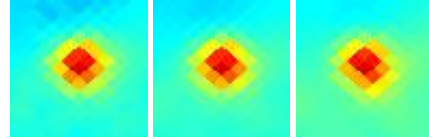
G296.49-15.77 J1055-771
