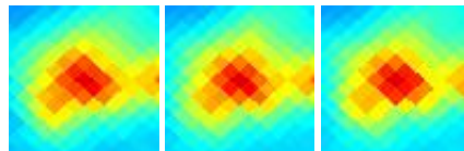
G000.92-20.16 J1914-368
