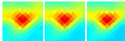
G099.97+14.76 J2033+653
