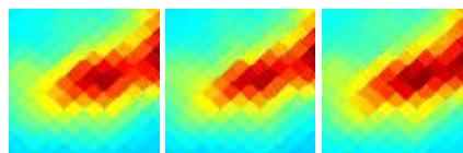
G166.99-15.34 J0413+297
