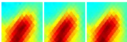
G005.03+19.07 J1649-141
