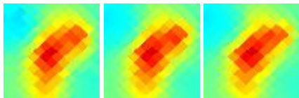
G217.46-13.78 J0609-101
