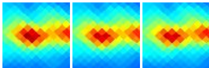
G217.13-12.54 J0613-093
