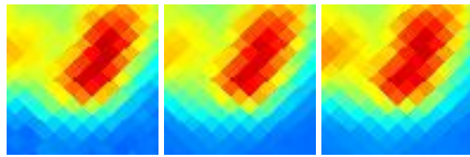
G359.91-00.09 J1745-290
