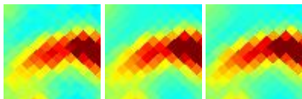
G216.01-15.94 J0559-098
