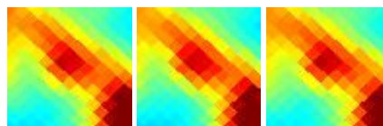
G173.18-09.12 J0453+293
