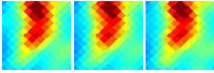
G339.65+09.27 J1609-390
