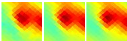
G206.05-08.36 J0609+022
