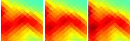
G278.32-00.93 J0946-547
