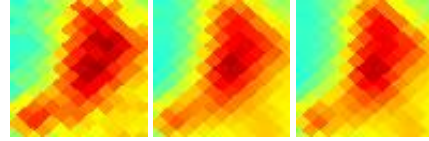
G294.98+03.35 J1150-585
