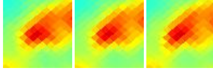
G254.00+08.36 J0850-308
