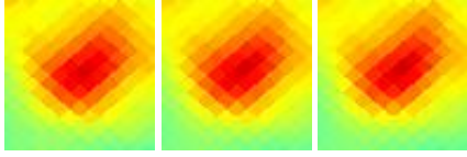
G251.93-01.17 J0807-347
