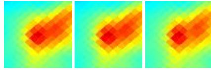
G092.83-11.03 J2205+419
