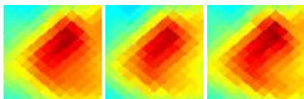
G003.07+09.95 J1716-209
