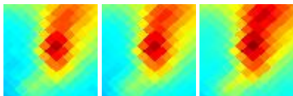
G129.22+15.17 J0240+766
