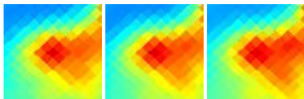
G303.85-14.16 J1307-770
