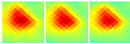
G133.48+09.02 J0254+693
