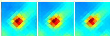
G220.67-01.86 J0658-077
