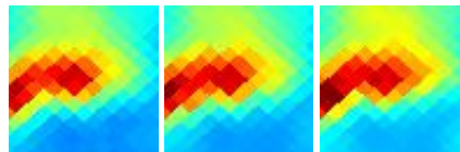
G200.34-10.97 J0549+059
