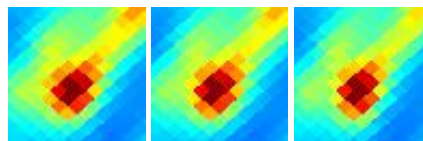
G094.08+09.46 J2041+575
