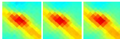
G215.92-15.32 J0601-095
