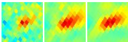
G127.22-02.25 J0126+603
