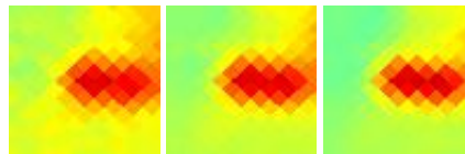
G098.89+14.01 J2033+640
