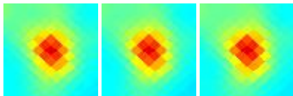
G110.41+11.52 J2213+704
