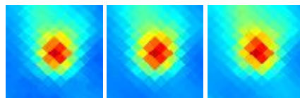
G003.14+08.19 J1722-218
