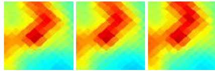
G093.36-12.06 J2211+414
