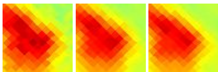
G017.22-01.47 J1827-146
