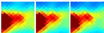
G001.23+09.91 J1711-224
