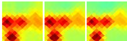
G097.84+15.32 J2018+638
