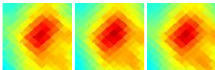
G006.04+36.74 J1554-028
