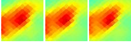
G253.49-01.26 J0811-360
