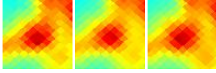
G339.10+15.44 J1546-348
