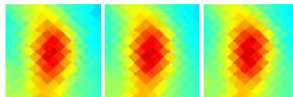
G222.23+01.21 J0712-077
