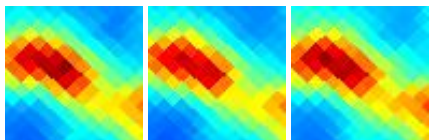
G170.77-08.51 J0448+315
