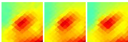
G203.20-11.20 J0553+033
