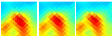
G303.68-15.32 J1305-781
