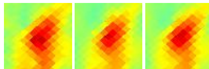
G172.92-16.74 J0426+246
