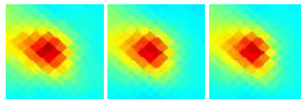
G096.30+10.01 J2048+596
