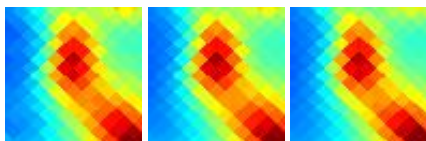
G303.15-13.78 J1255-766
