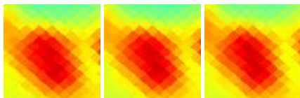
G096.59+10.29 J2047+600
