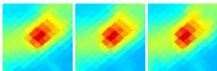
G095.29-09.66 J2212+444
