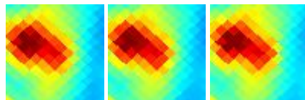
G205.57-08.25 J0608+027
