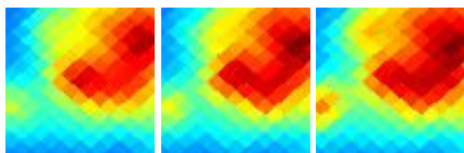
G202.30-08.91 J0600+052
