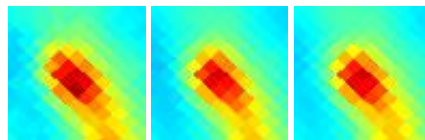
G174.99-04.83 J0514+304
