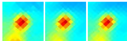
G112.60+08.53 J2252+689
