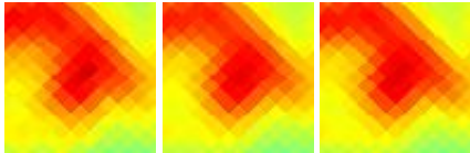
G296.52-15.67 J1056-770
