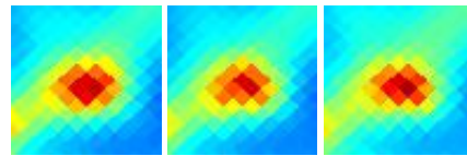
G354.81+00.35 J1731-331
