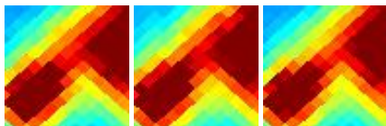
G194.80-03.41 J0605+144
