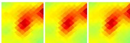
G264.22+06.05 J0914-399
