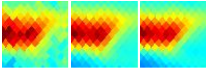
G156.92-09.72 J0357+405
