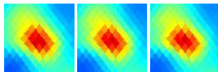
G210.89-36.53 J0435-142
