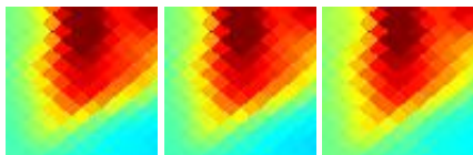
G266.74+04.98 J0919-425
