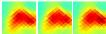
G003.73+18.30 J1648-156
