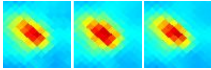
G359.31+17.03 J1642-197
