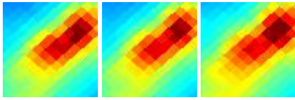
G341.19+06.48 J1625-400
